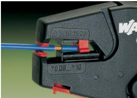
Quickstrip 10. Зачистка провода.
